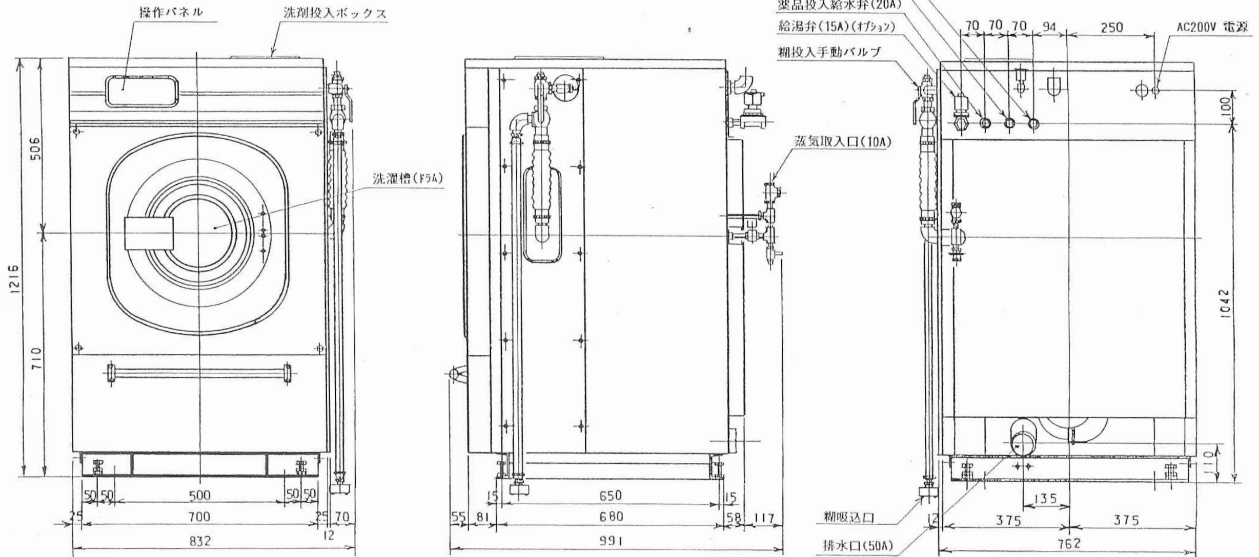
WN70 自動水洗機外観図
