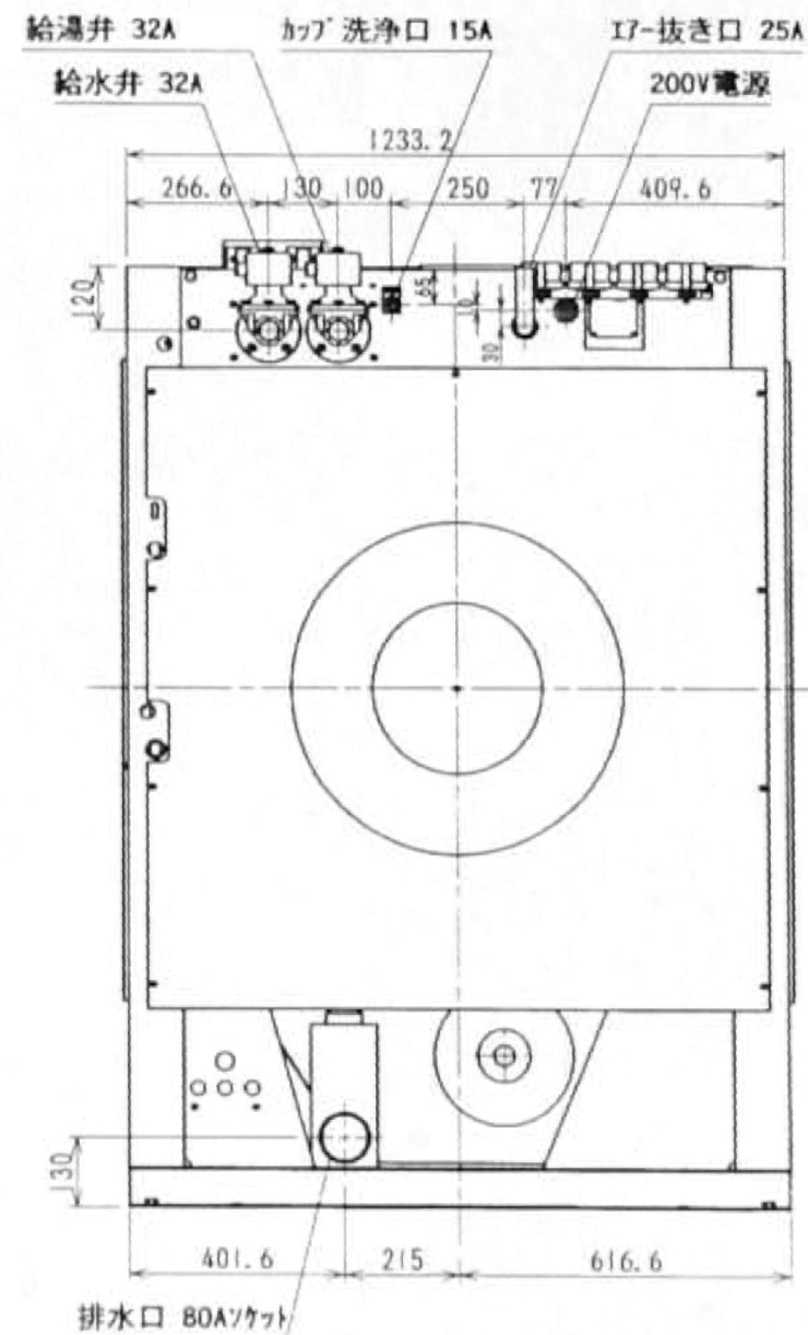
WN351施設用 外観図
