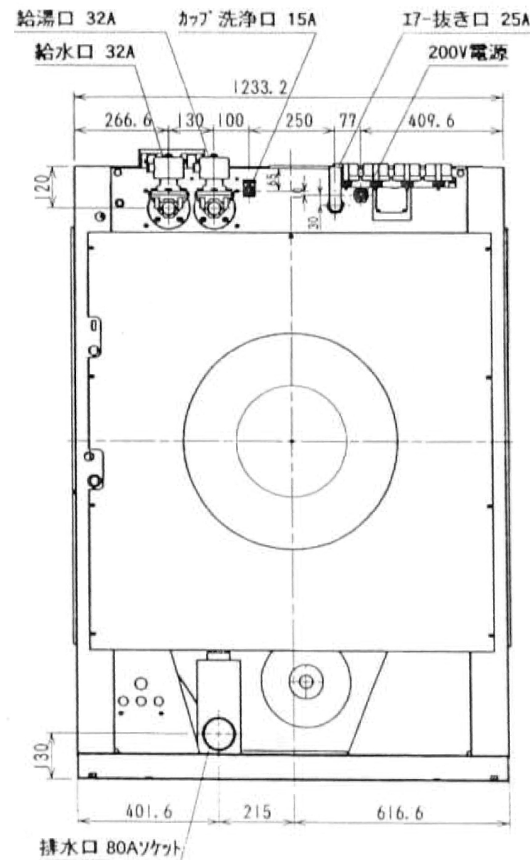
WN301施設用 外観図
