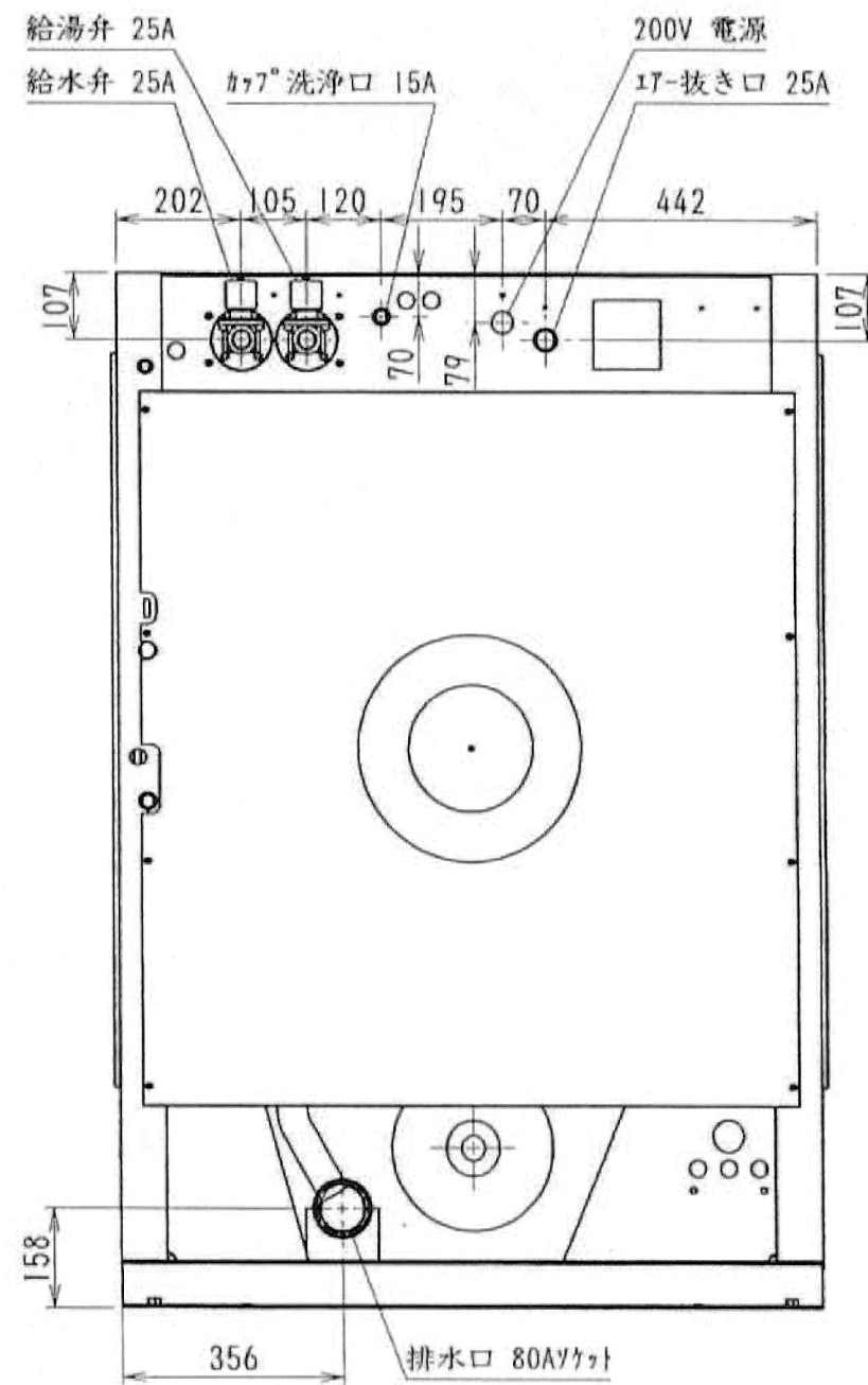
WN221 外概観図
