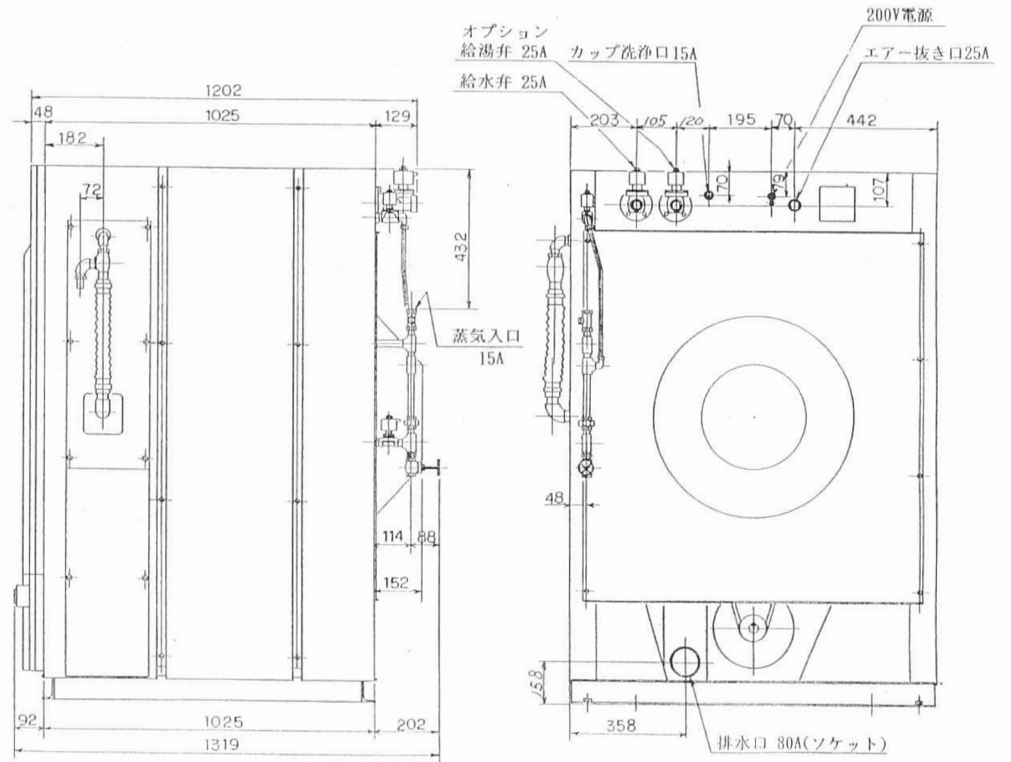
WN221D 外観図
