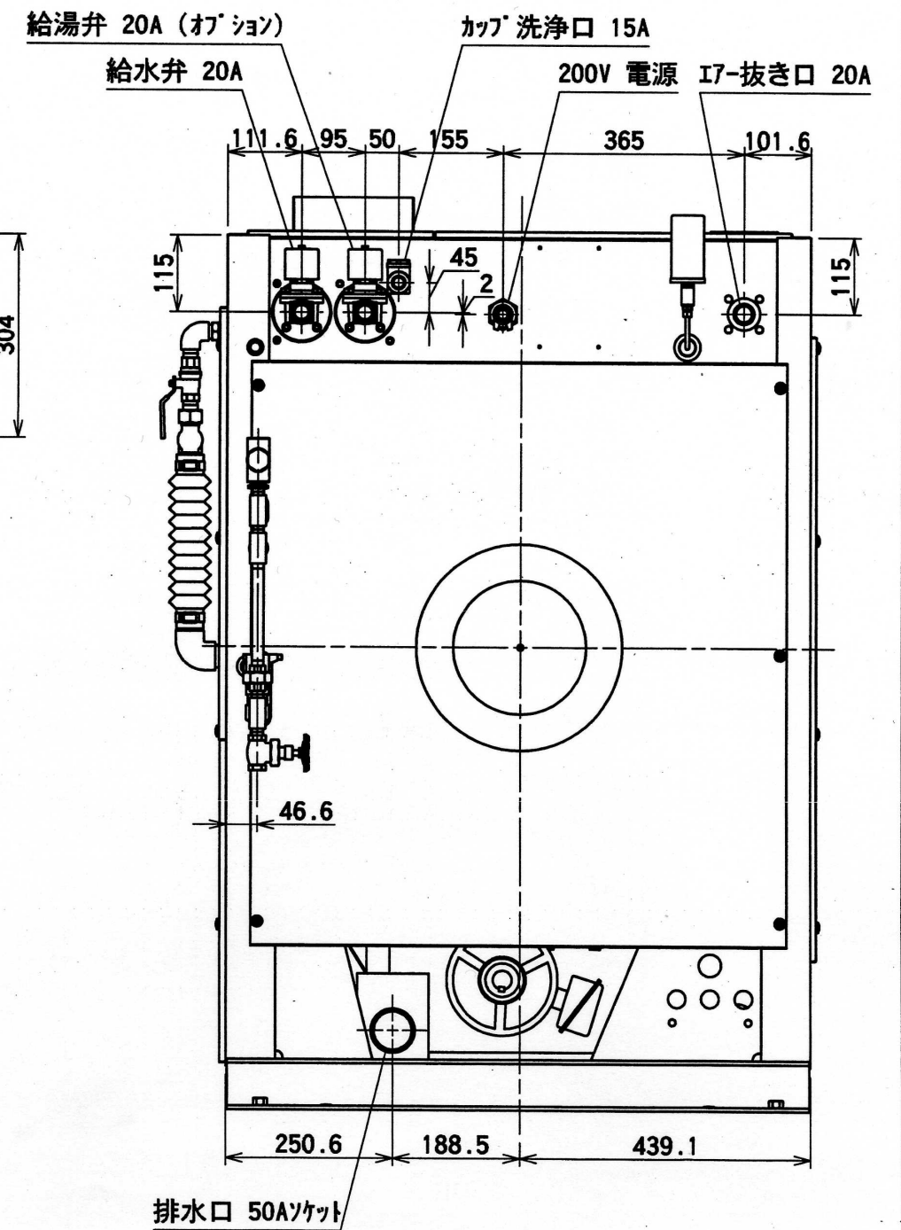
WN101 外観図
