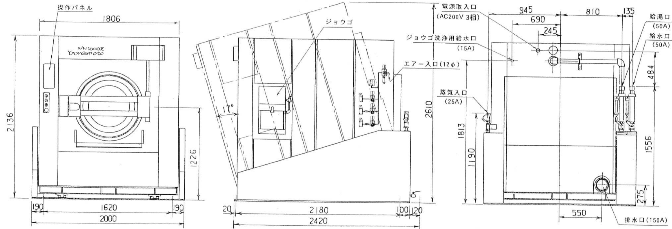
WN1000Z 外観図
