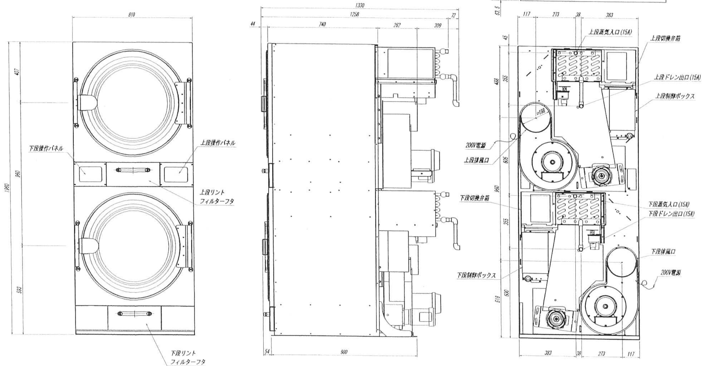
VS101W 外観図
