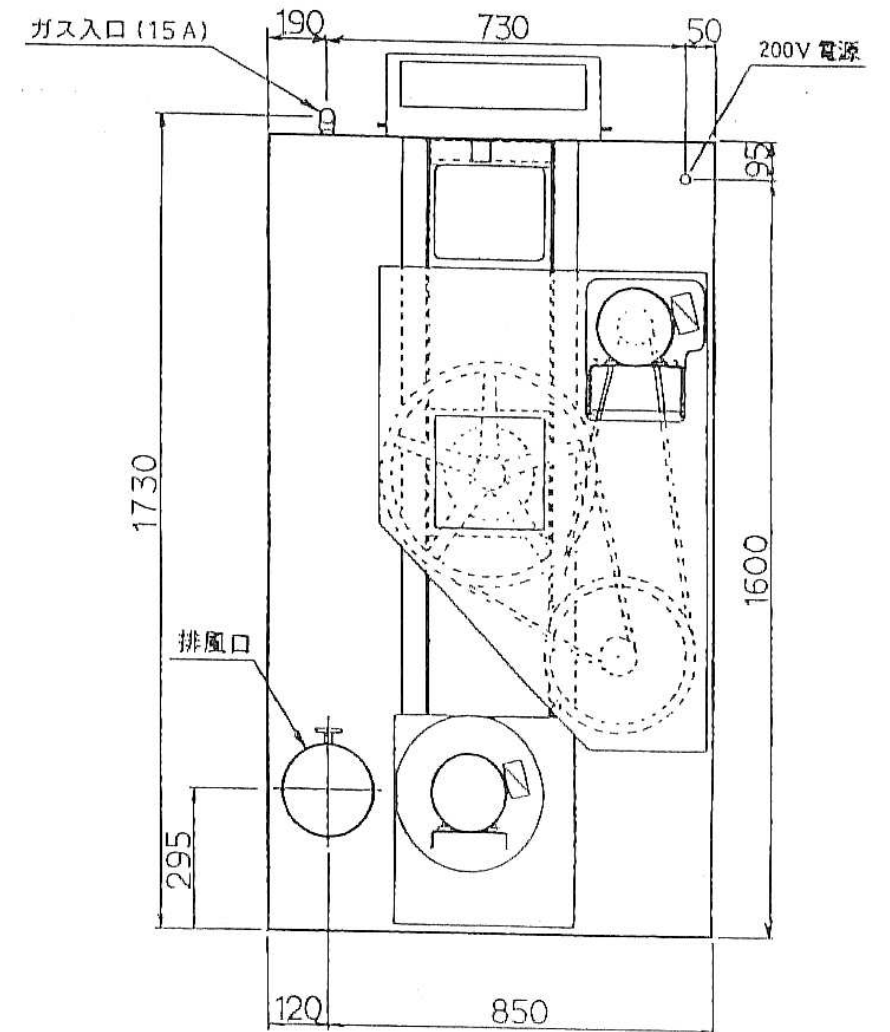
VG221 外観図
