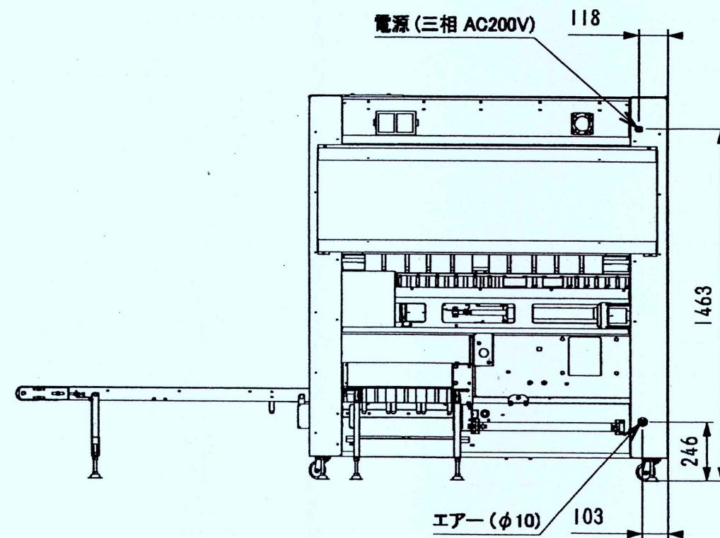
FT10F3外観図
