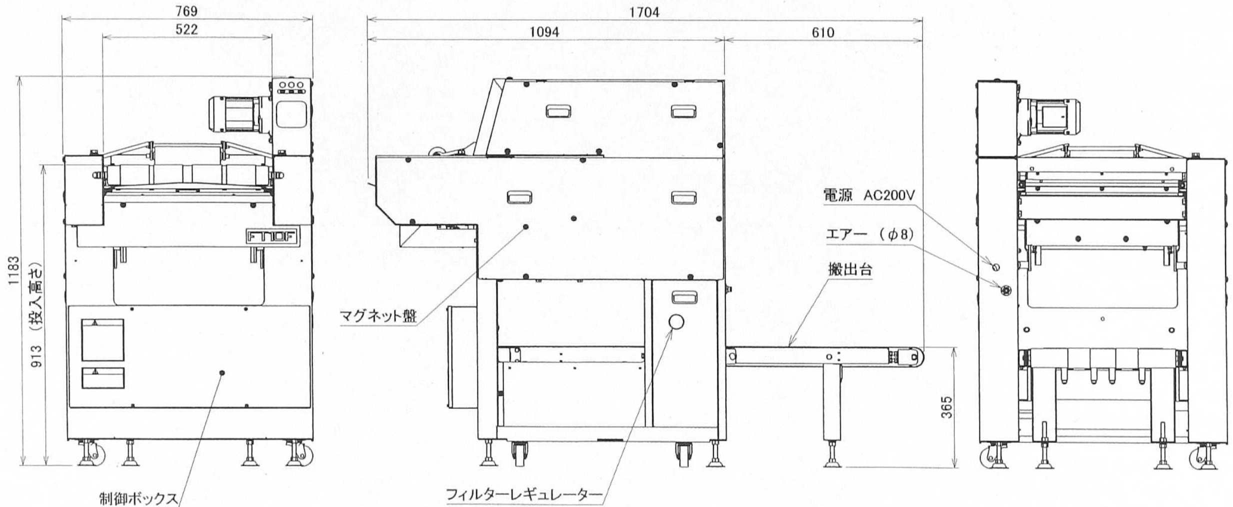
FT10F外観図
