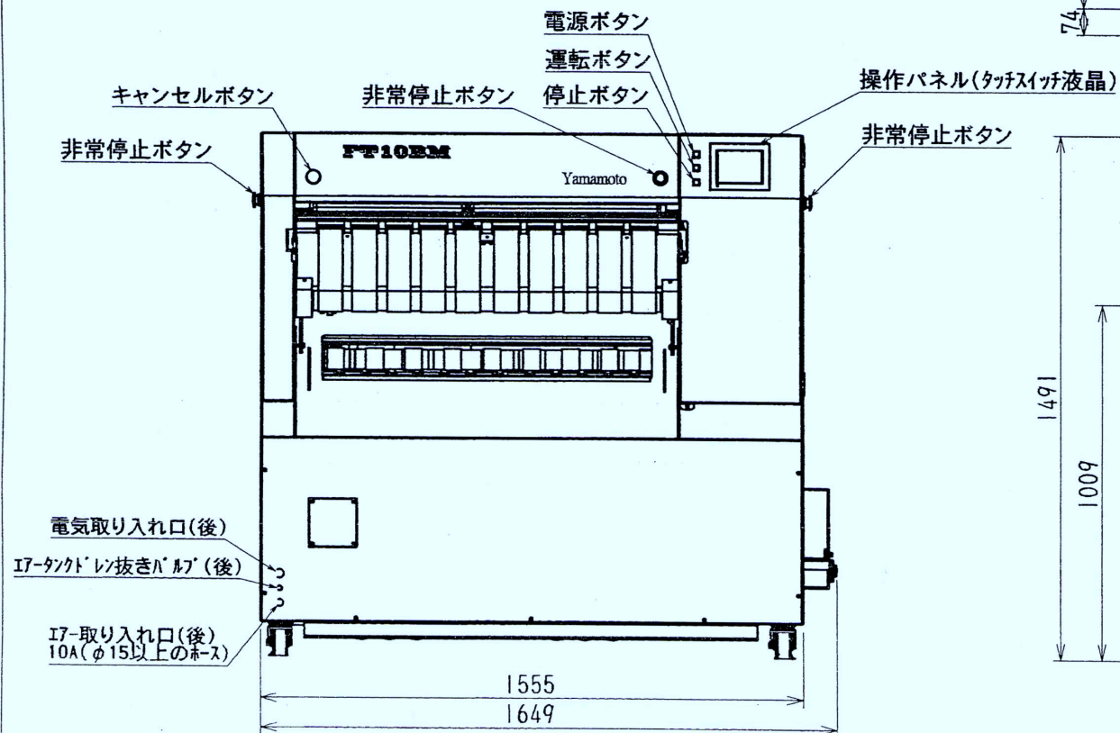
正面図
