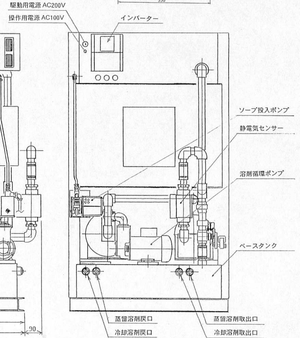
DO100FD 外観図
